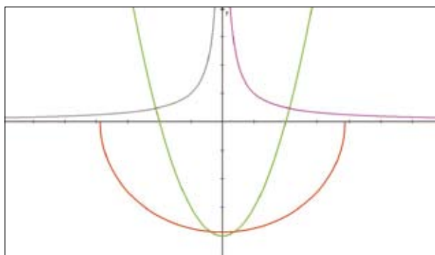
Figur 4: Konvekse kurver
